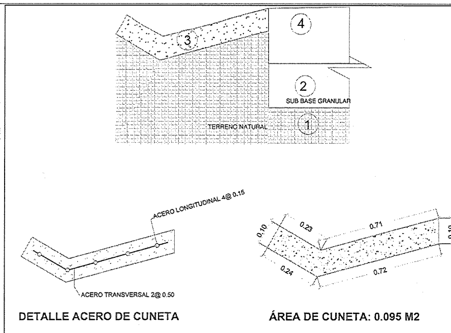
Ilustración 2 Detalle de las cunetas a construir Fuente: Archivos del proyecto – Plano Diseños Estructura de Pavimento
