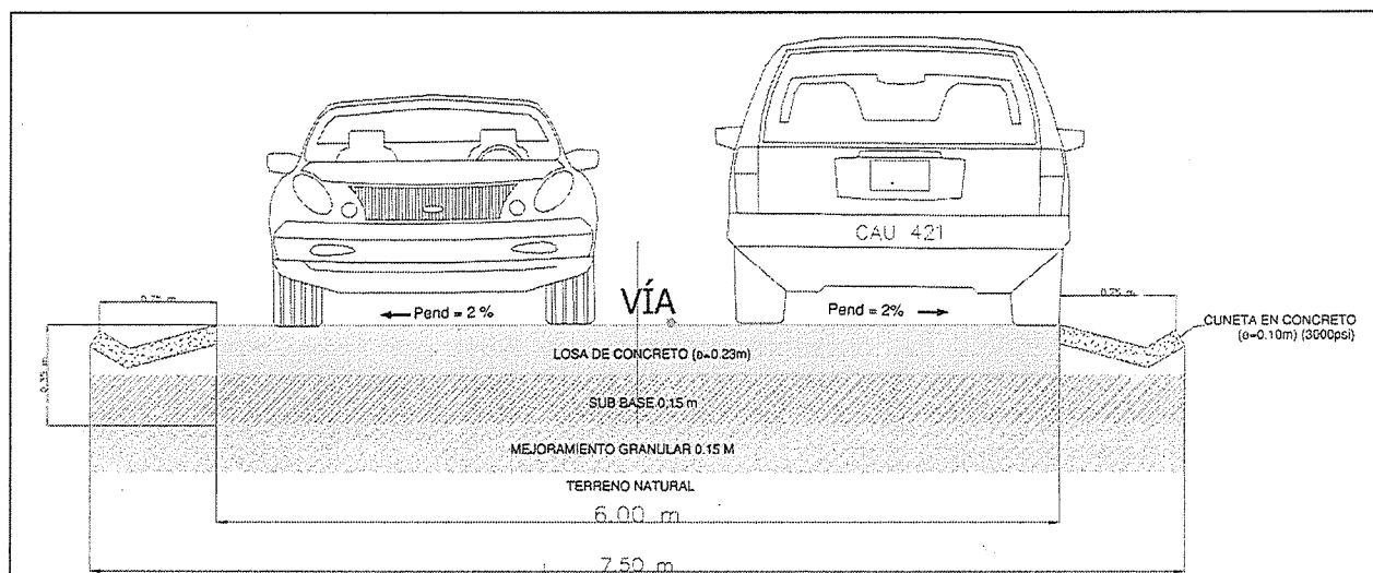
Ilustración 1 Detalle de la estructura de pavimento a construir Fuente: Archivos del proyecto – Diseño de Pavimento
